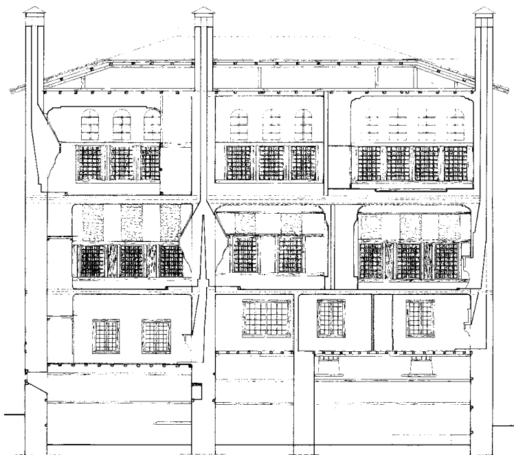
Τομή Α-Α
