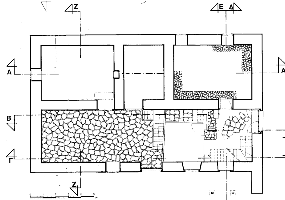
Κάτοψη μεσοπα- τώματος
