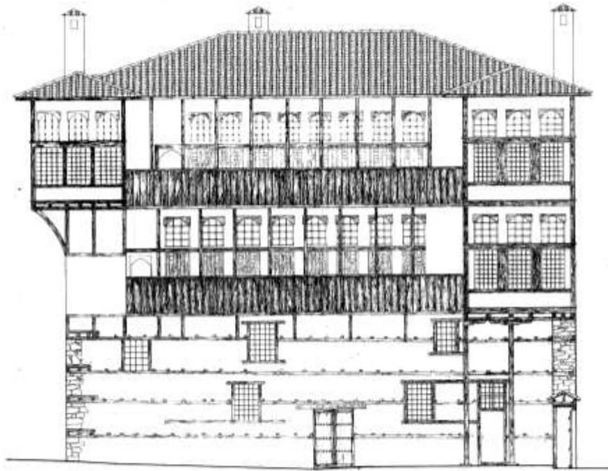
Βόρεια όψη
