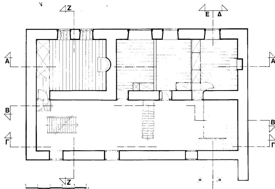
Κάτοψη ισογείου
