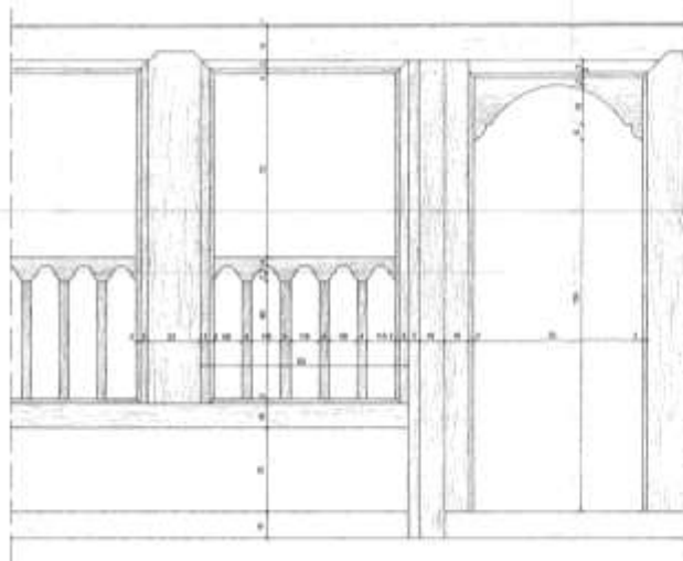
Ανοίγματα Βόρειας Όψης Α6
