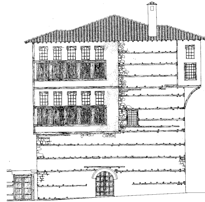
Δυτική όψη
