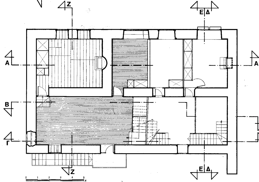
Κάτοψη μεσοπα- τώματος
