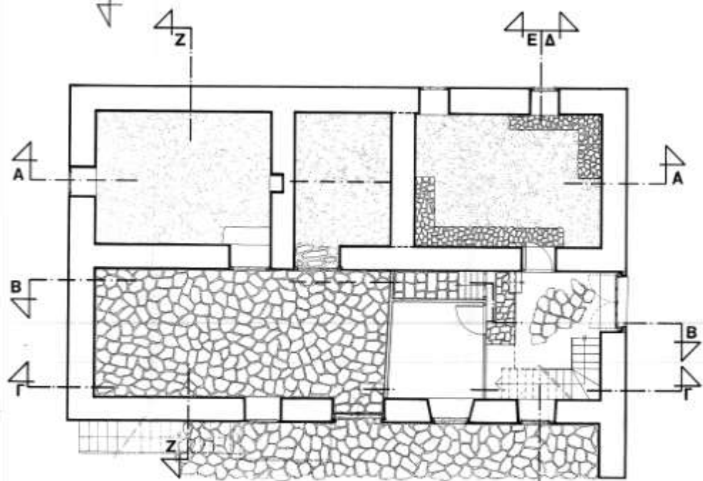
Κάτοψη ισογείου
