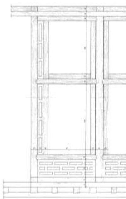
Κατασκευαστική λεπτομέρεια ΒΘ Α1
