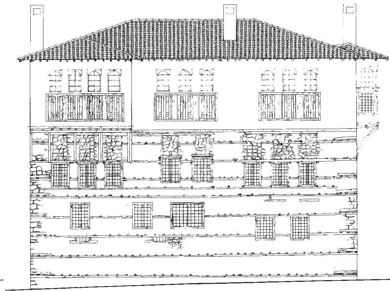
Νότια όψη
