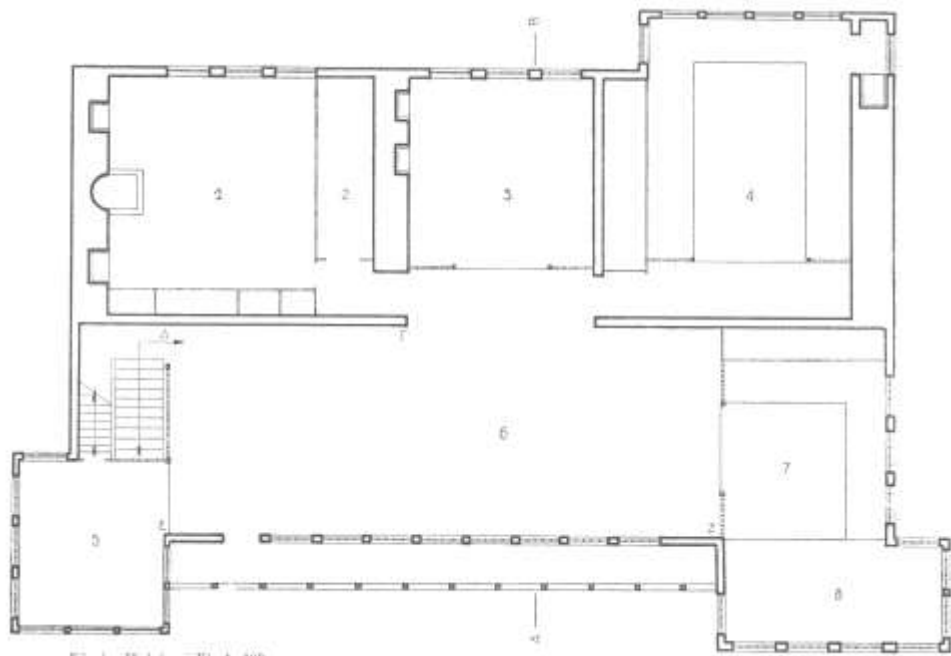
Κατάψας Β' όρόφου Κλ. 1 : 100
