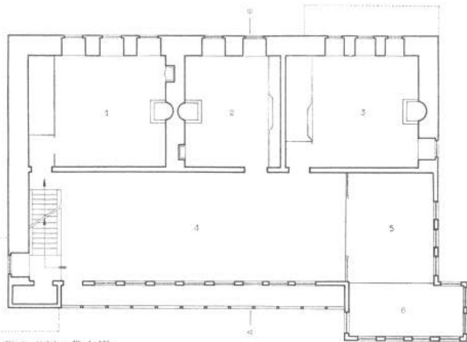
Κατάψας Α' όρόφου Κλ. 1 : 100
