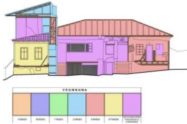
Σχ. 6 Βόρεια όψη. Οικοδομικές φάσεις
