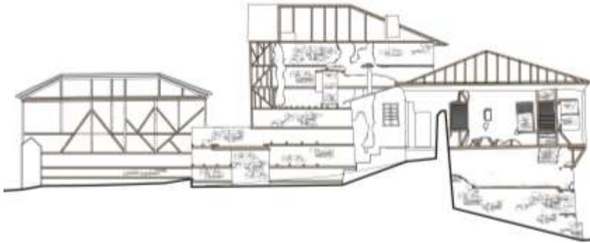
Σχ. 13 Δυτική όψη. Αποτύπωση
