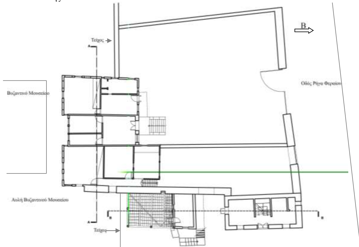
Σχέδιο 1. Κάτοψη συγκροτήματος. Αποτύπωση υφιστάμενης κατάστασης
