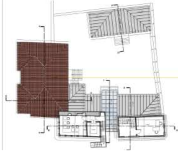
Σχ. 10 Στάθμη 3. Πρόταση. Μοναδικό δάπεδο του ΝΑ κτηρίου (αριστερά) τοποθετείται το καθιστικό του κυλικείου και δίπλα η κουζίνα. Στον όροφο του ΒΑ κτηρίου ένα ακόμα γραφείο
